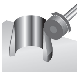
Möglichkeiten zum Schleifen eines Hohlsliffs für besondere Anwendungen
